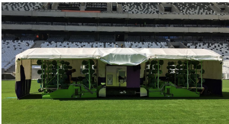
Rys. 17 Montaż zszywanej trawy hybrydowej
